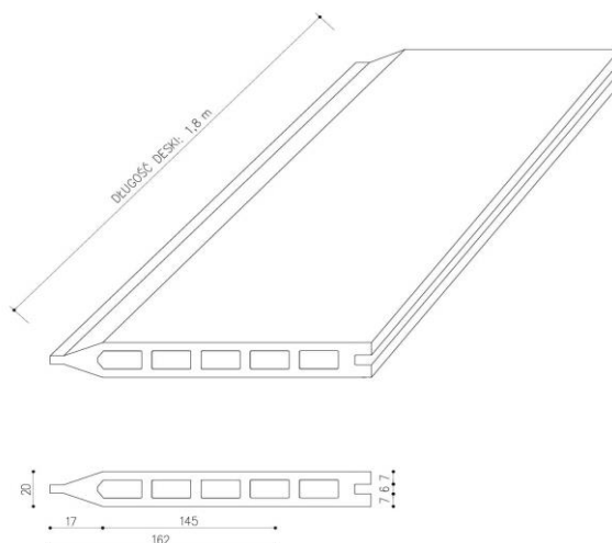
DESKA OGRODZENIOWA STANDARD 1800 x 162 x 20 mm
